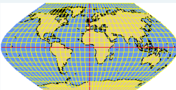
PUTNINS5 hyperbolic
